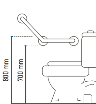
Barre de relevage coudée
